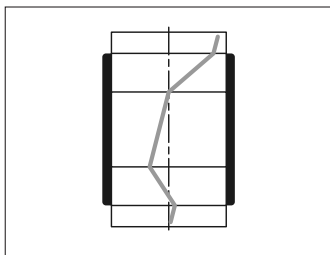
Fig 9 Poulies à trois désalignements combinés
