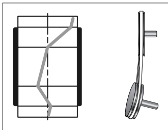
Рис 8 Отображение комбинации трех видов несоосности
