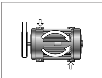
Fig 12 Alignement angulaire horizontal
