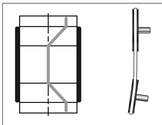
Рис 6 Отображение горизонтальной угловой несоосности
